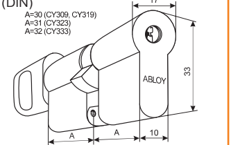
ABLOY® CY323 (CY309) ABLOY® CY333 (CY319) СТАНДАРТ EUROPROFILE (DIN) класс 2 класс 4
