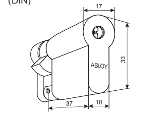
ABLOY® CY303 ABLOY® CY313 СТАНДАРТ EUROPROFILE (DIN) класс 2 класс 4
