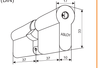
ABLOY® CY304 ABLOY® CY314 СТАНДАРТ EUROPROFILE (DIN) класс 2 класс 4
