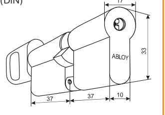
ABLOY® CY305 ABLOY® CY315 СТАНДАРТ EUROPROFILE (DIN) класс 2 класс 4
