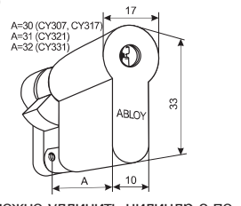
ABLOY® CY321 (CY307) ABLOY® CY331 (CY317) СТАНДАРТ EUROPROFILE (DIN) класс 2 класс 4
