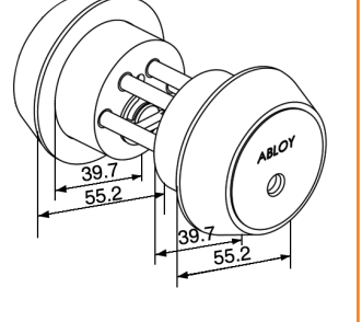
ABLOY® CY203 ABLOY® CY205 класс 4
