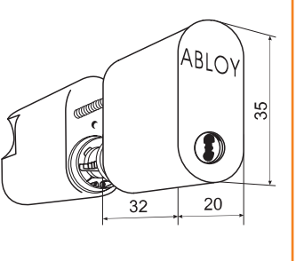
ABLOY® CY202 класс 2
