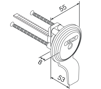
ABLOY® CY053 (5190) ABLOY® 5190 класс 2
