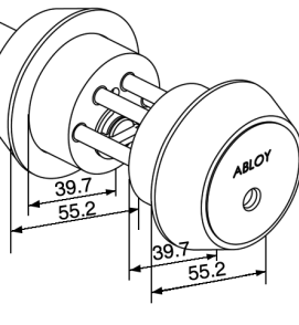
ABLOY® CY204 класс 4
