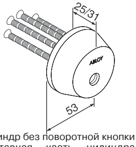
ABLOY® CY016 класс 3
