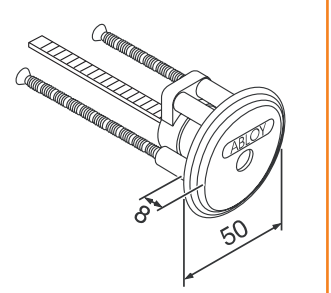
ABLOY® CY027 (5150) класс 2
