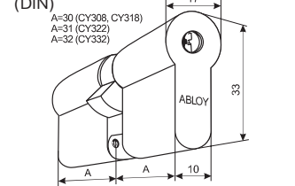
ABLOY® CY322 (CY308) ABLOY® CY332 (CY318) СТАНДАРТ EUROPROFILE (DIN) класс 2 класс 4
