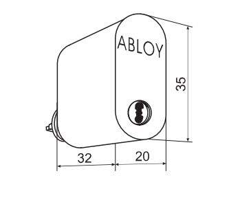
ABLOY® CY201 класс 2
